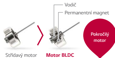
Střídavý motor
